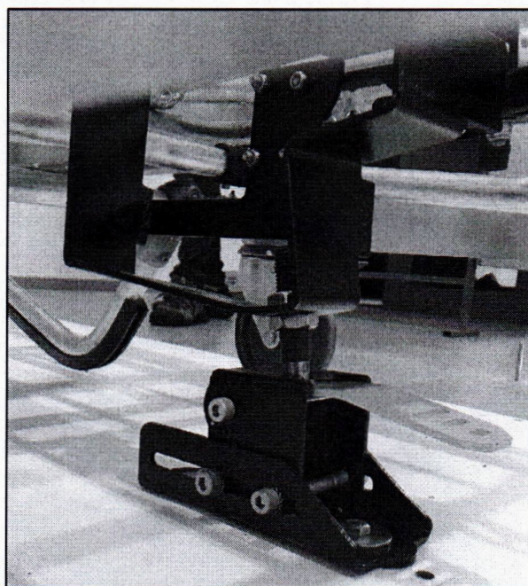
Figura 6 – Sistema de retenção traseiro após os ensaios
