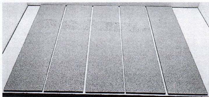
Figura 5: Corpos de prova utilizados para ensaio de inflamabilidade horizontal – NT246735.
