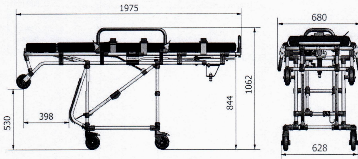
Figura 02 – Maca Armada
