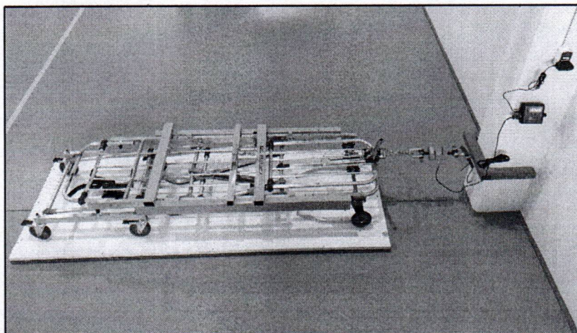
Figura 4 – Ensaio de tração frontal
