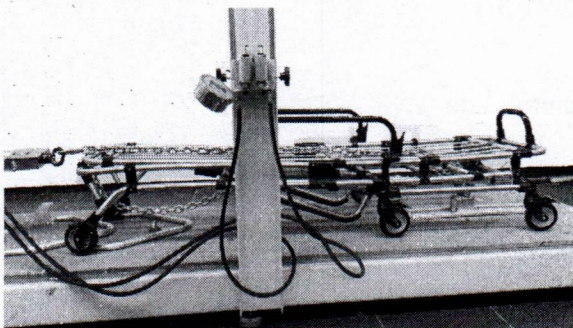
Figura 06 – Ensaio de tração frontal
