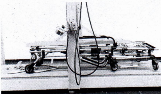
Figura 06 – Ensaio de tração vertical
