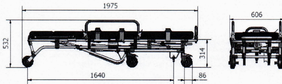
Figura 03 – Maca desarmada
