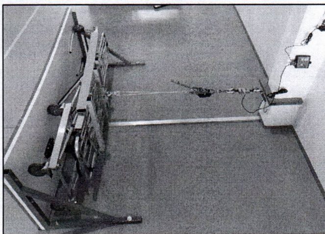
Figura 3 – Ensaio de tração vertical
