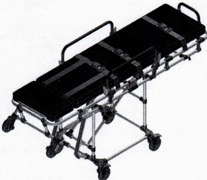
Figura 01 – Vista isométrica
