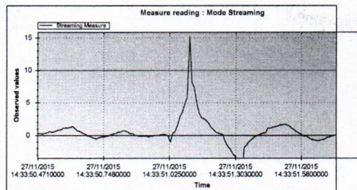
Figura 05 – Aceleração lateral
