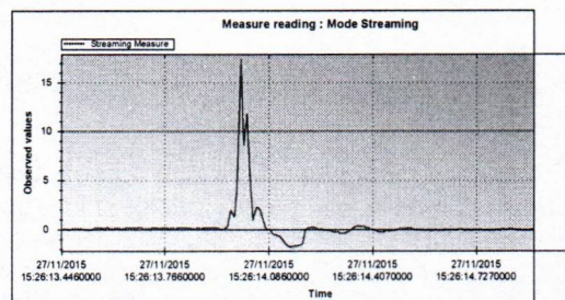
Figura 03 – Aceleração vertical
