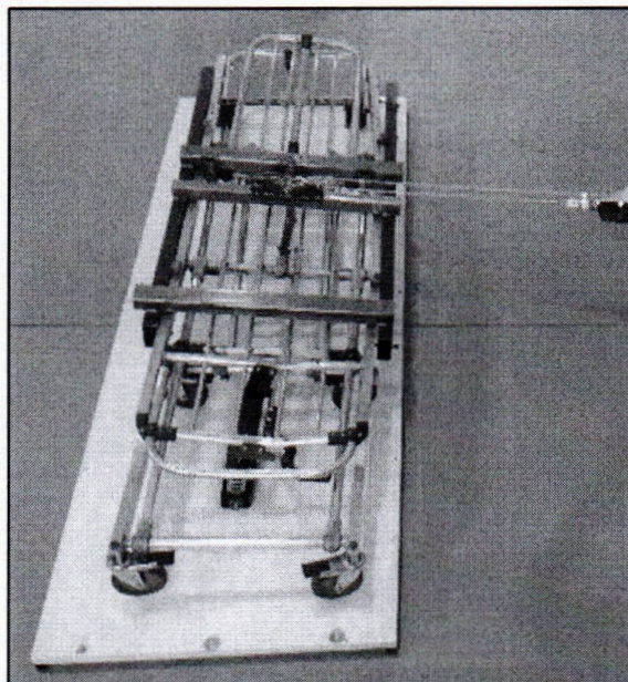
Figura 5 – Ensaio de tração lateral
