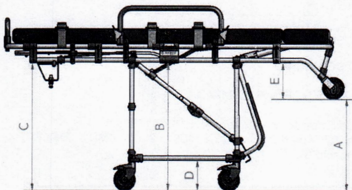
Figura 04 – Vista lateral
